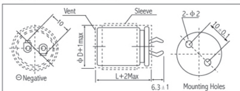
外形图尺寸表 Dimensions mm
